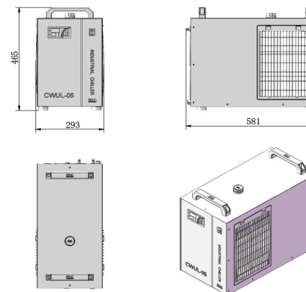
581(L)×293(W)×465(H)mm 3 ,
